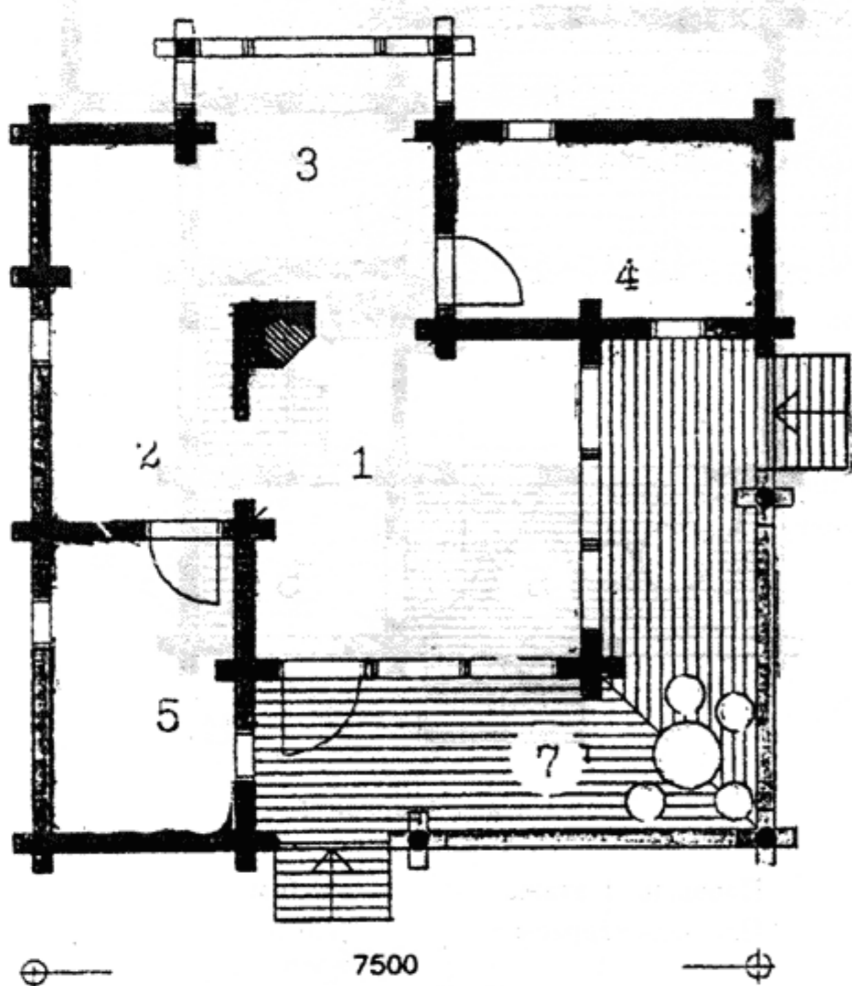
План 1 этажа
