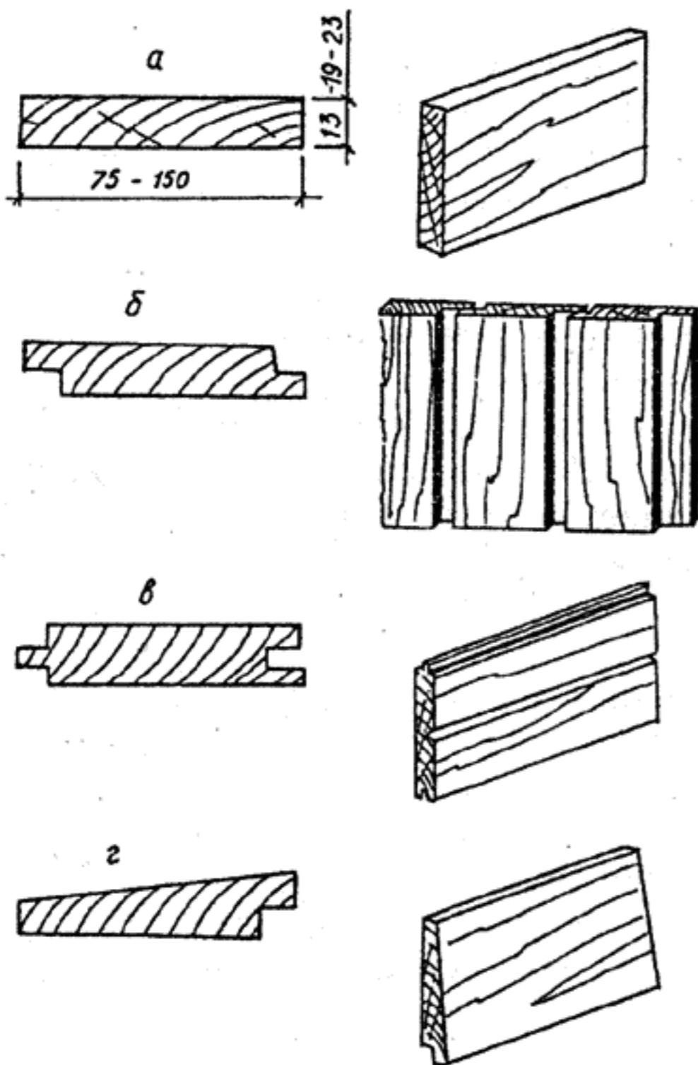
Отделочная доска:
