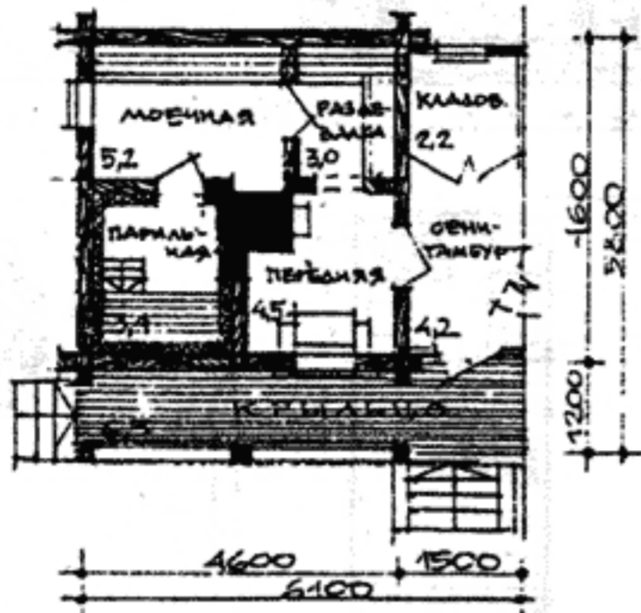
ПЛАН М 1:100
