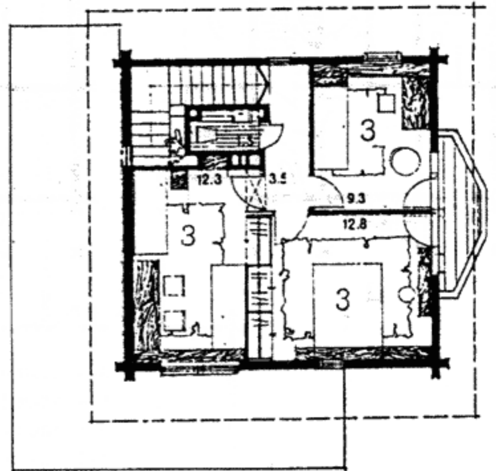
План 2 этажа
