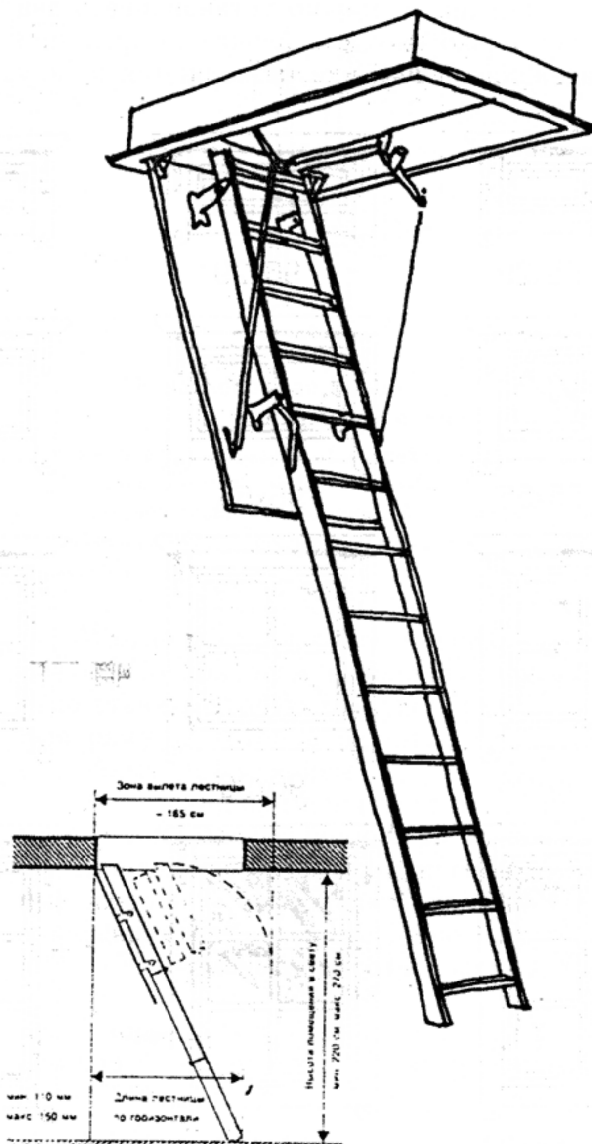
Складная стремянка. Фирма «Рото Франк» (Германия)
