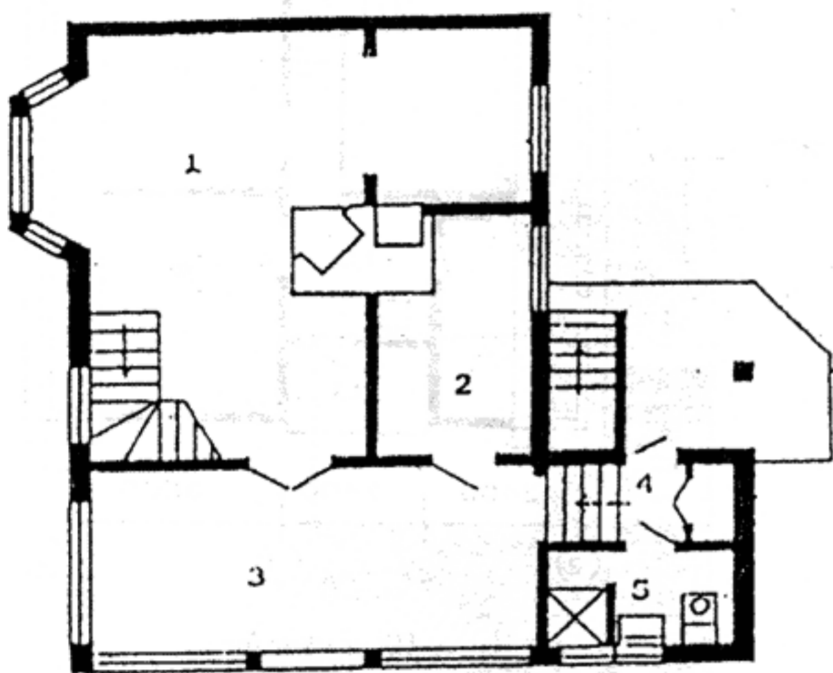
План 1 этажа
