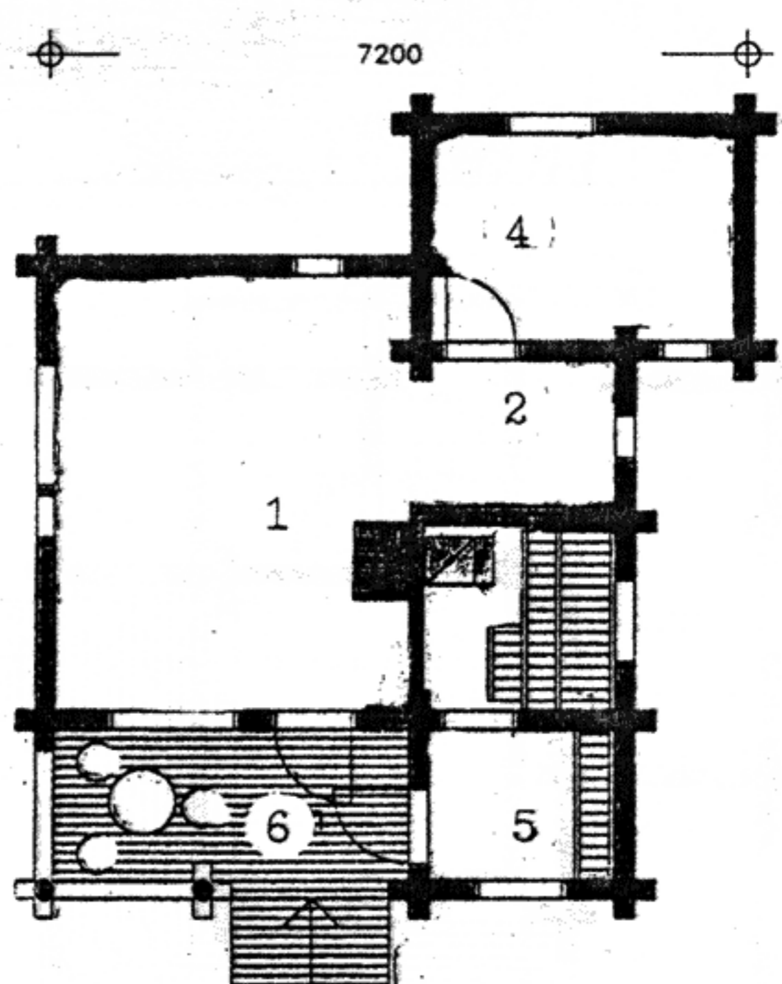
План I этажа (вариант)
