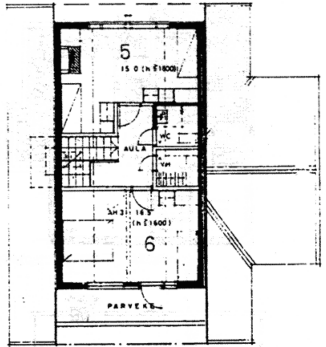
План мансарды
