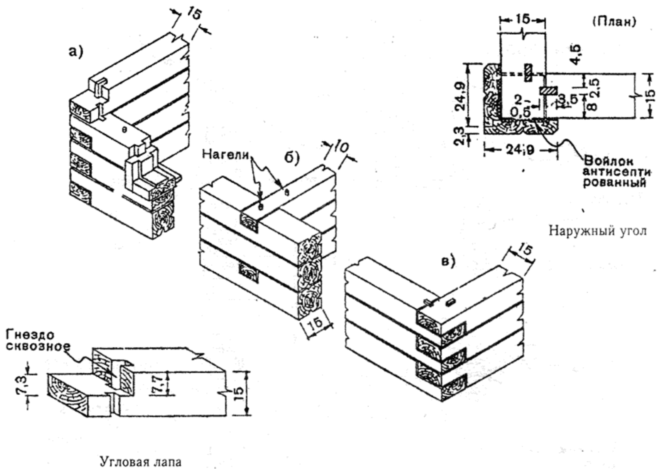
Сопряжение стен в полдерева
