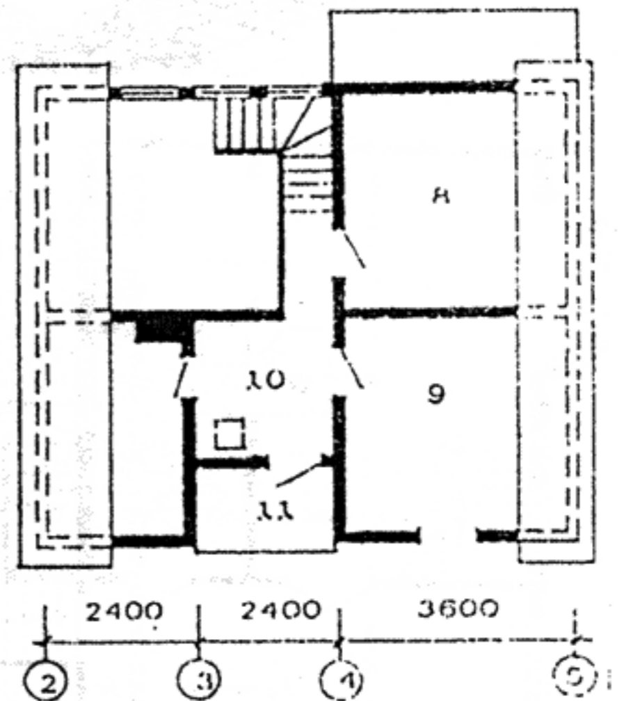
План мансарды
