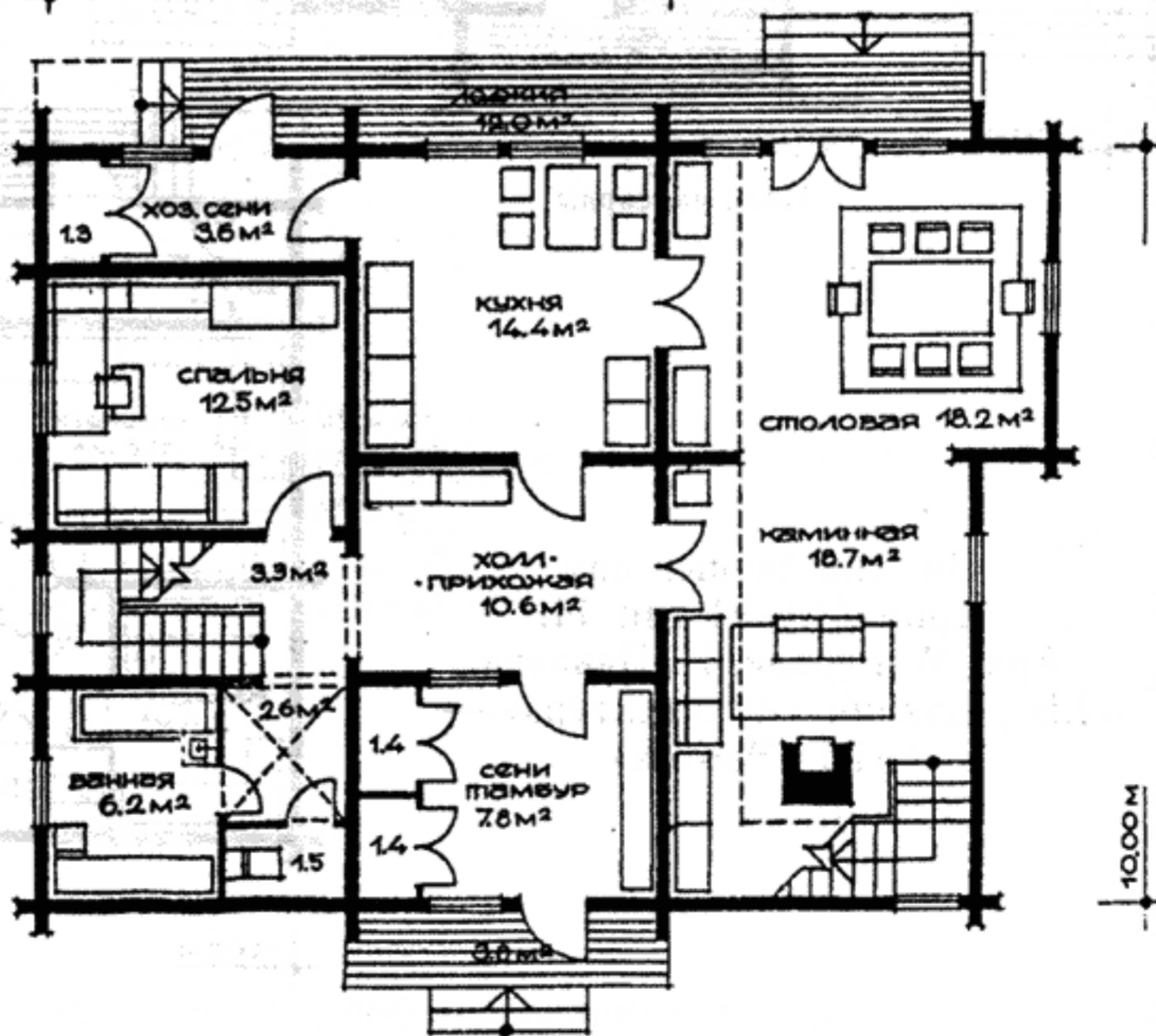
План 1 этажа
