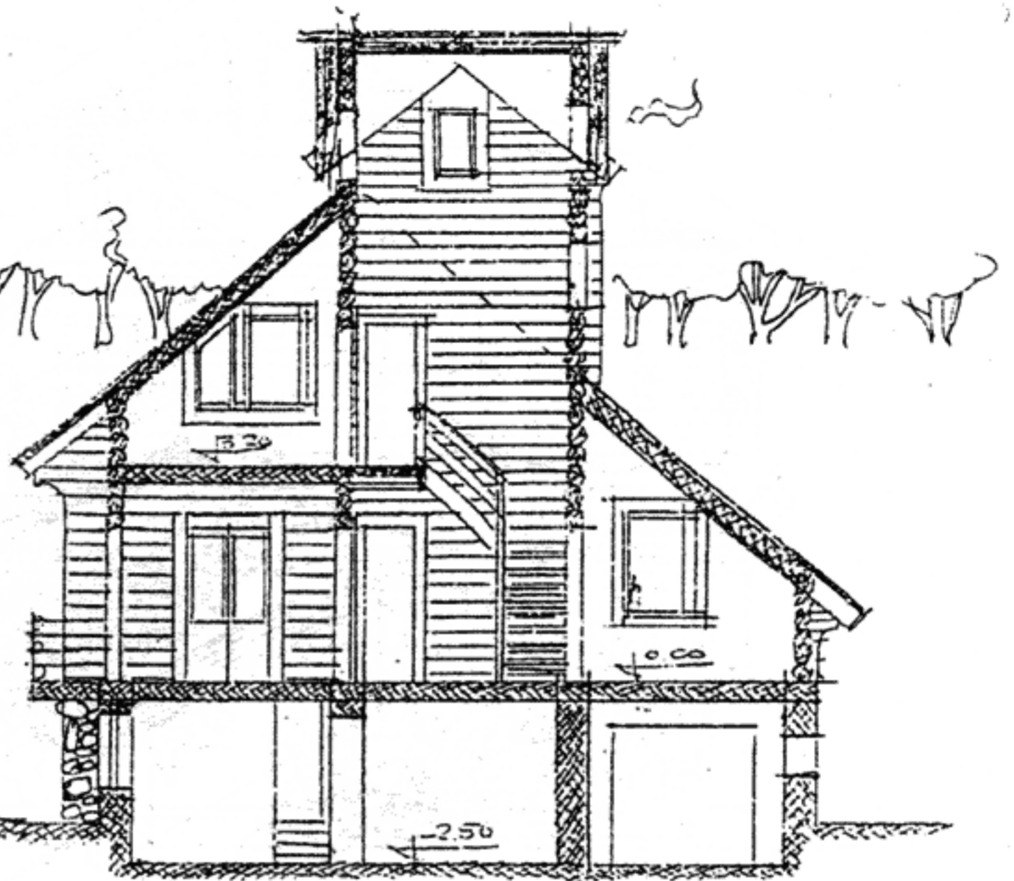
Разрез
