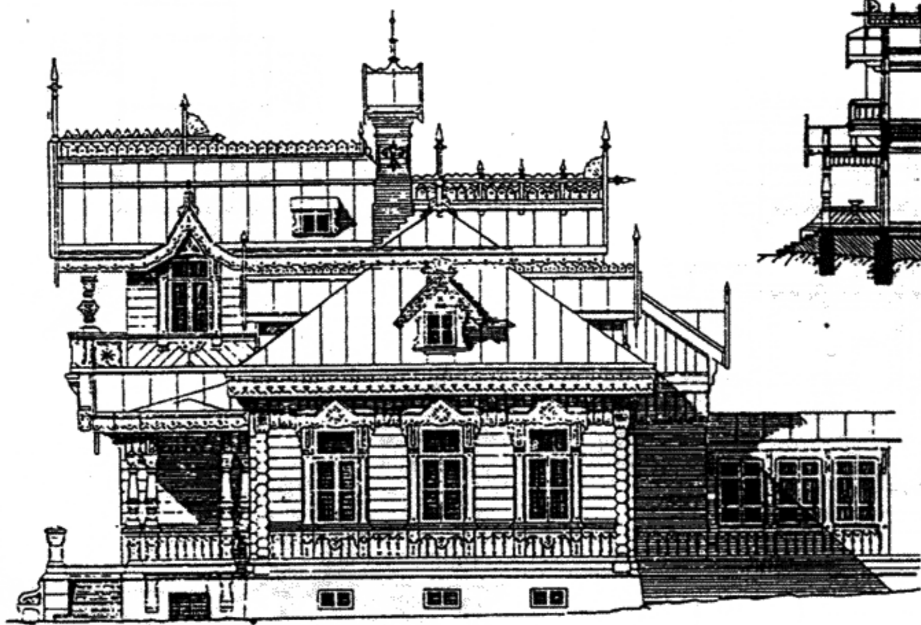
Боковой фасад
