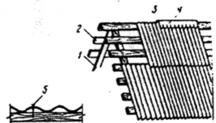
Кровля из асбестоцементных листов:
