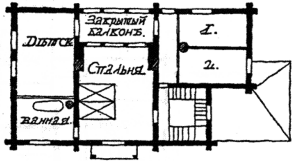
Планъ II эт.
