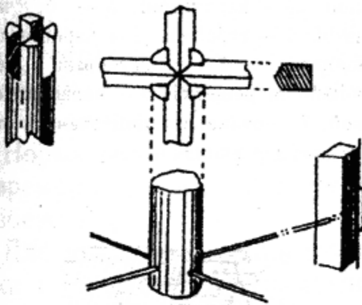
Узлы
