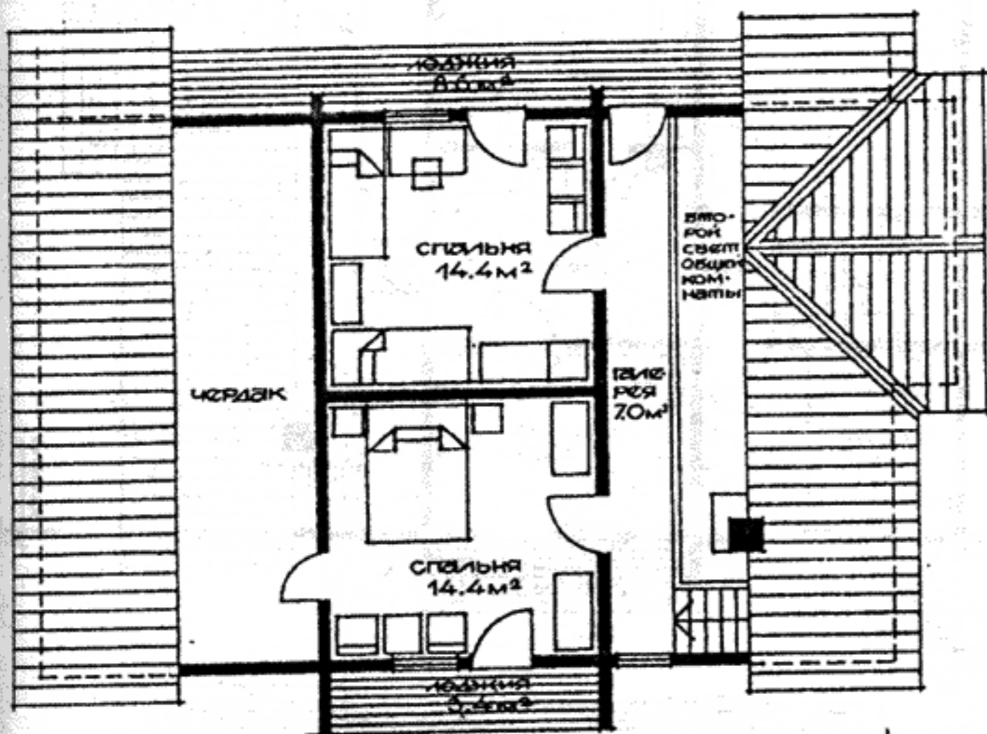
План мансарды
