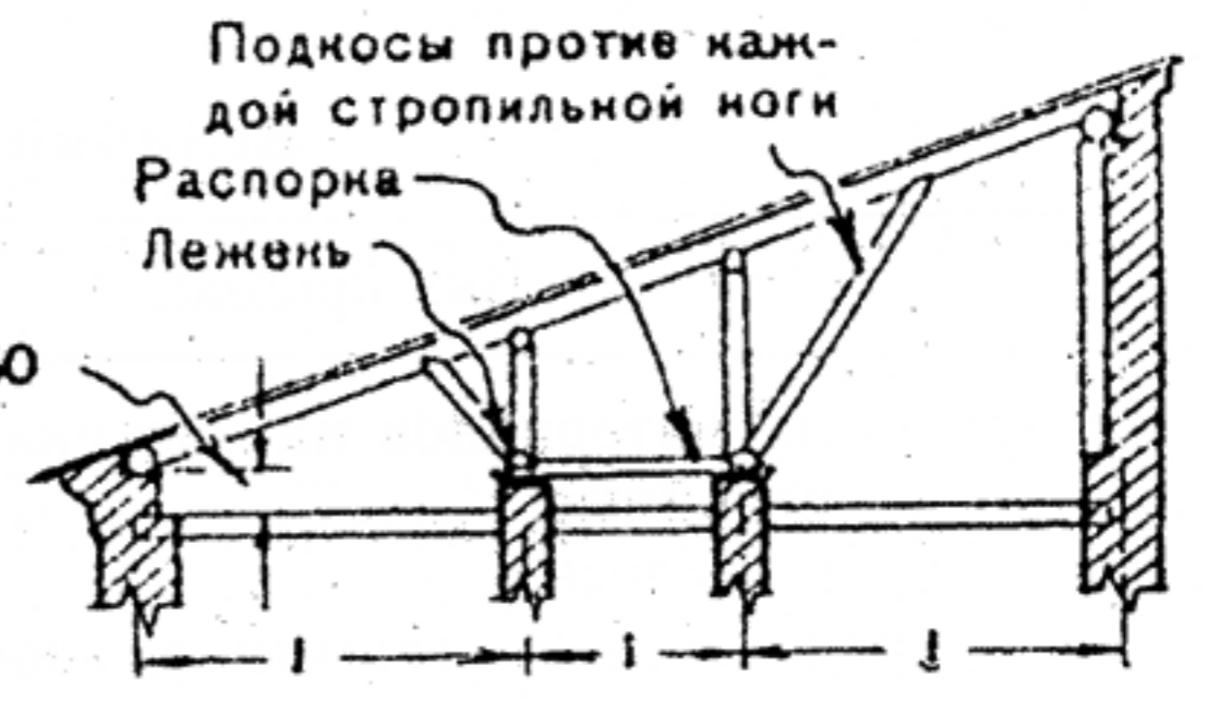
Схемы стропил односкатных кровель:
