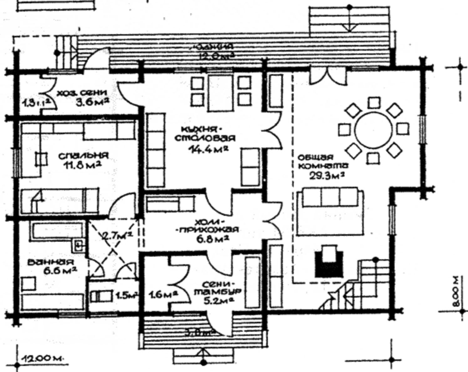
План I этажа
