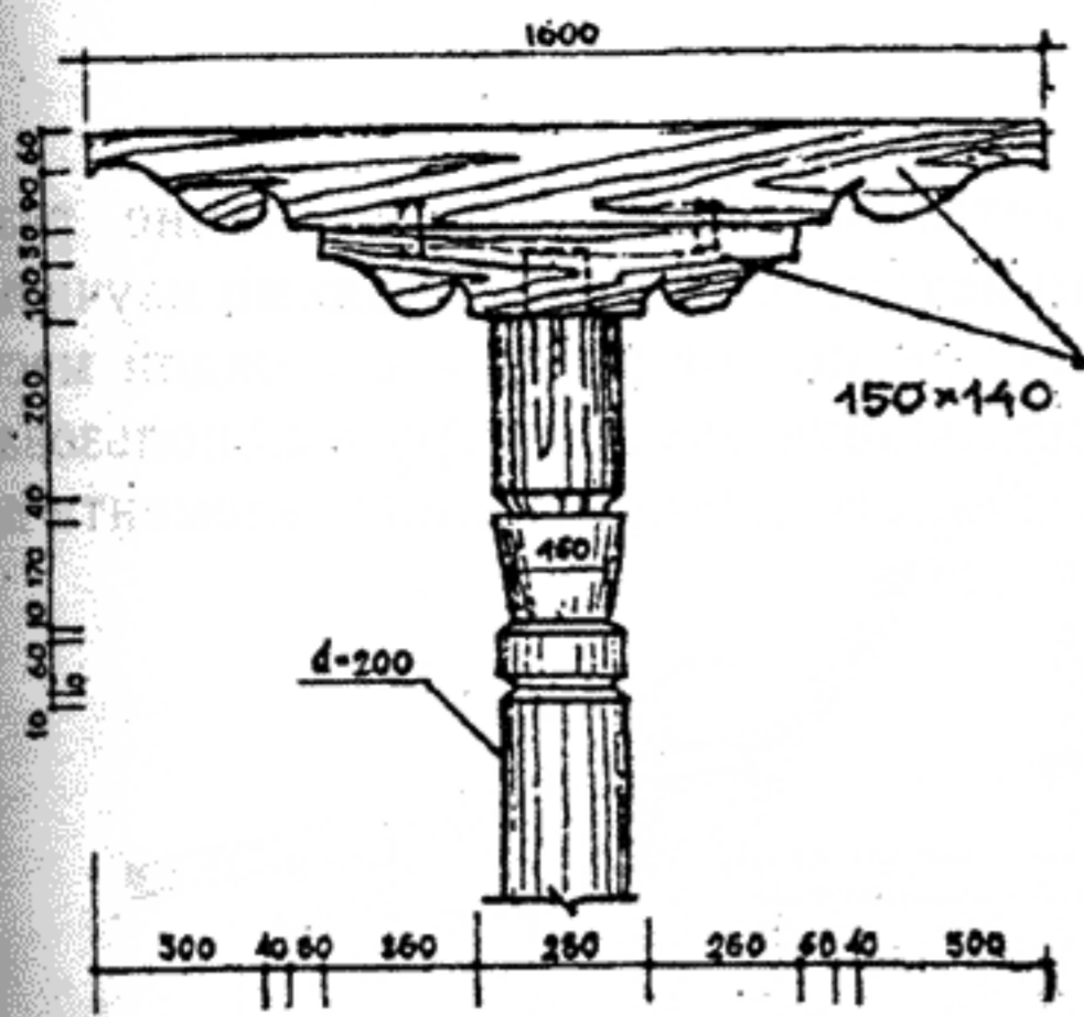
Деталь обшивки фронтона и лобовой доски
