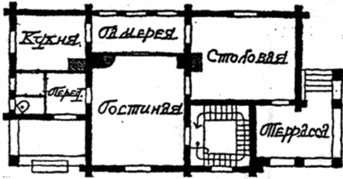
Планъ I эт.
