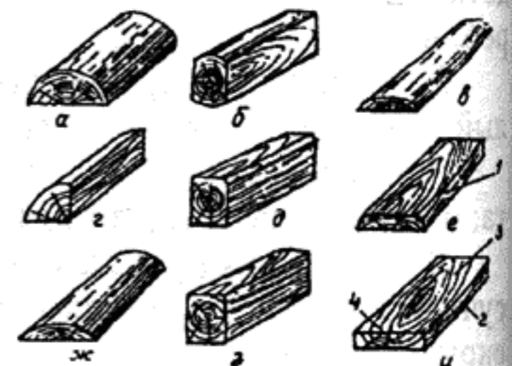
Виды пиломатериалов:
