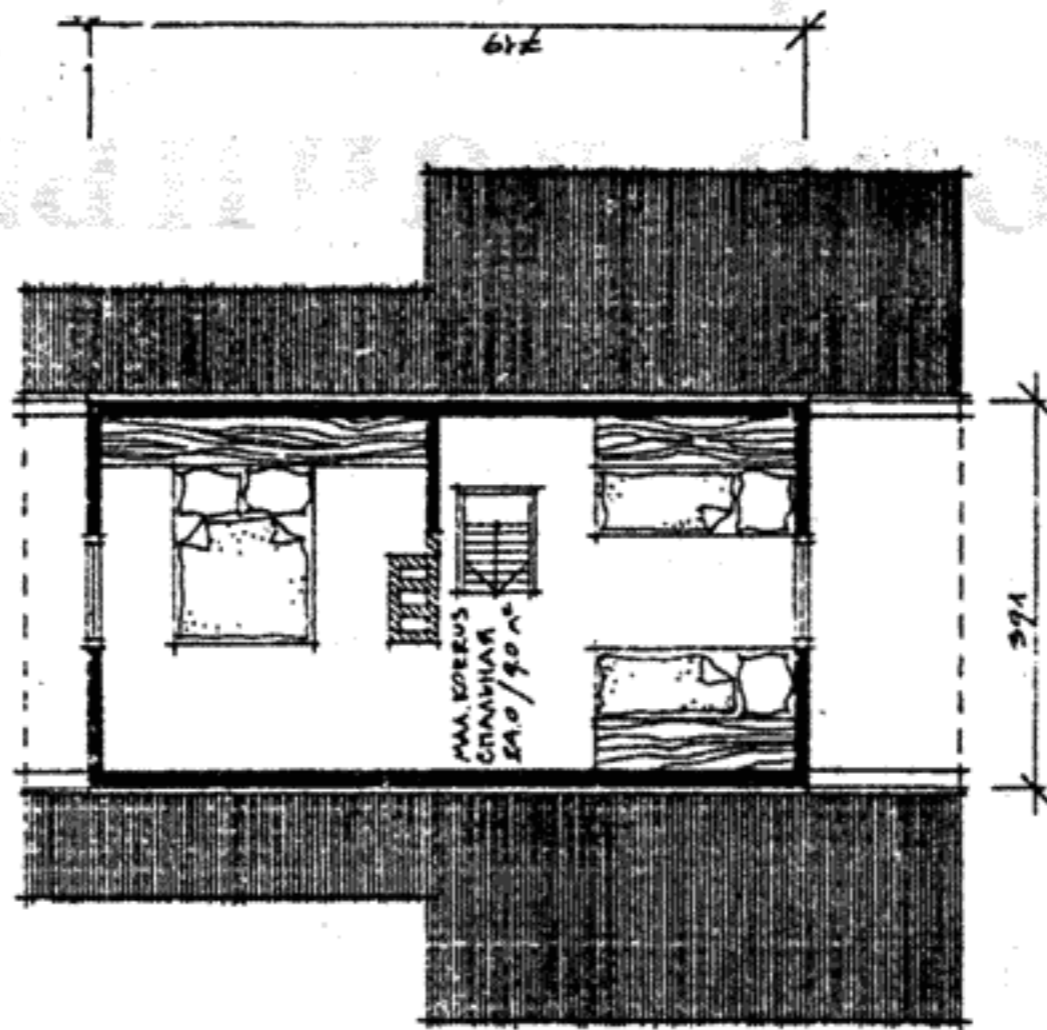
План мансарды
