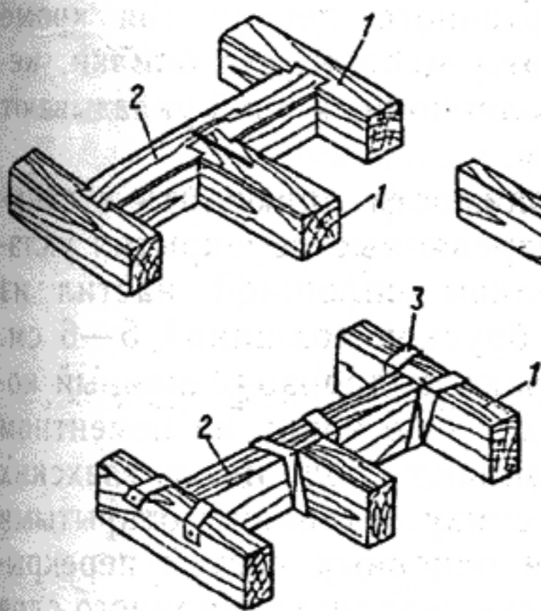
Крепление ригеля к балкам перекрытия:
