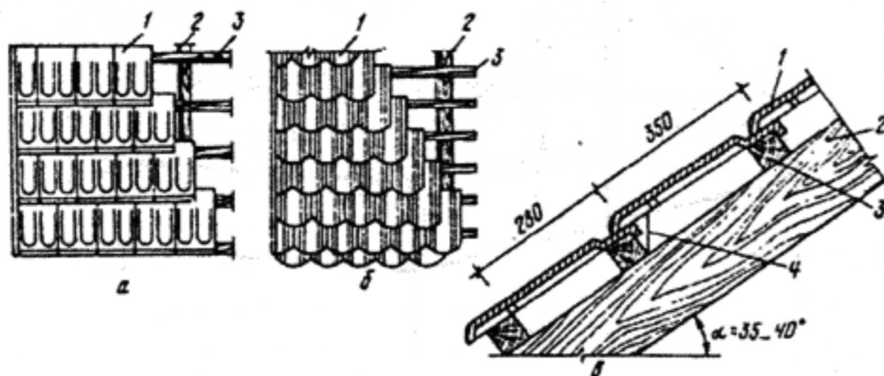
Черепичная кровля:
