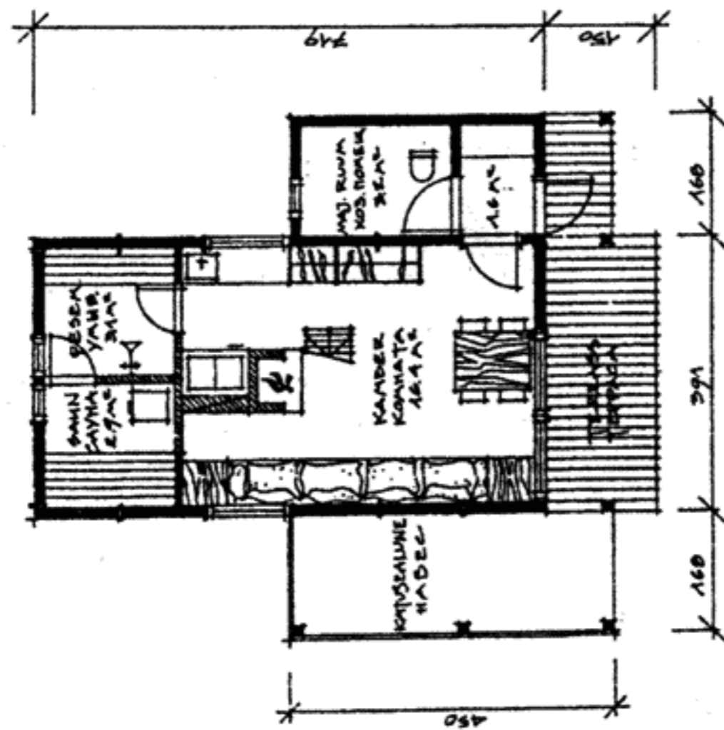
План 1 этажа
