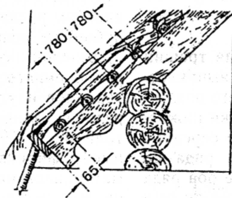
б) разрез
