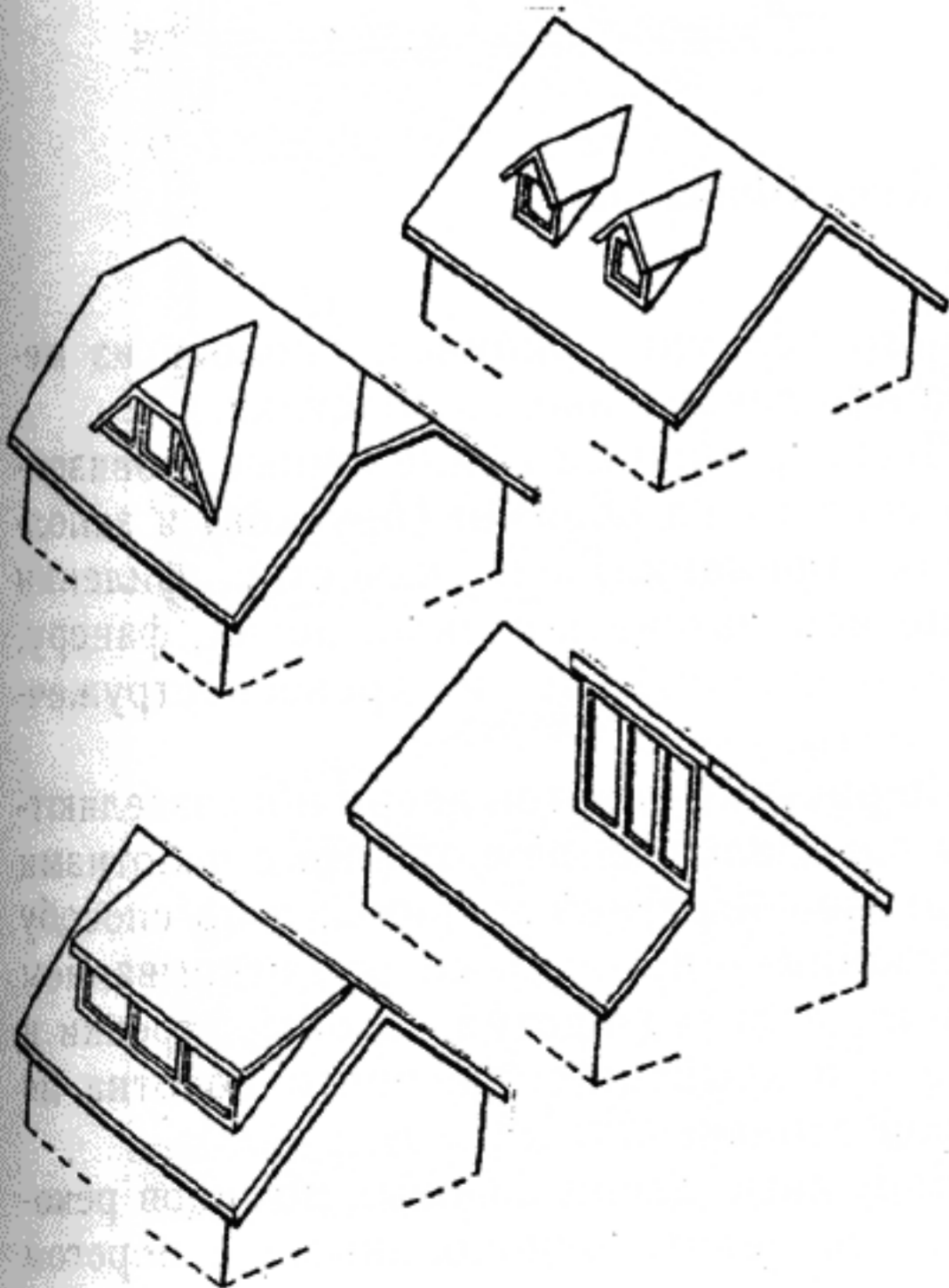
Окна в мансардной крыше
