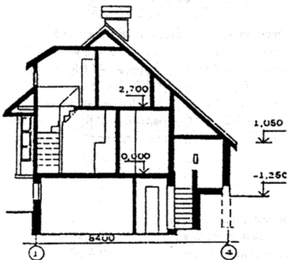
Разрез
