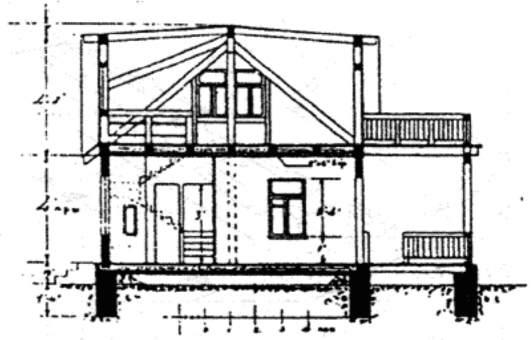
Разрез
