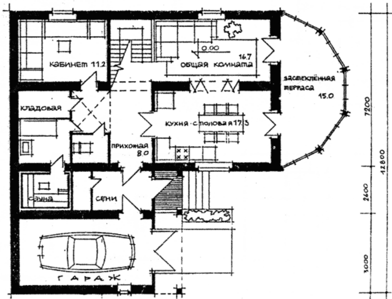
План 1 этажа
