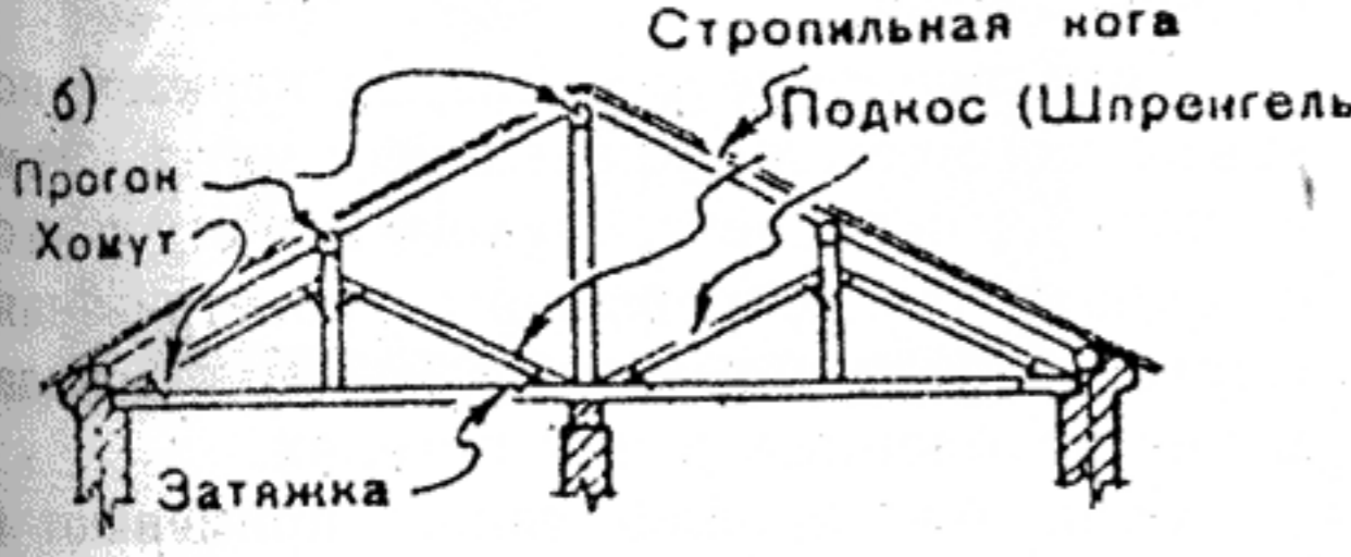
Элементы крыши
