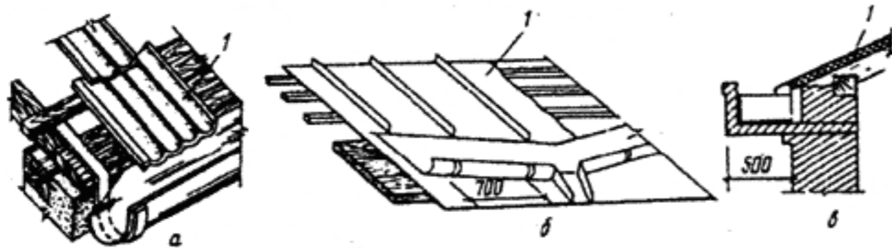
Устройство желобов для сброса атмосферных вод с крыши:
