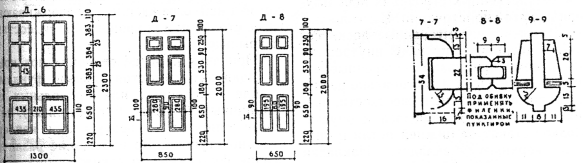
Двери внутренние
