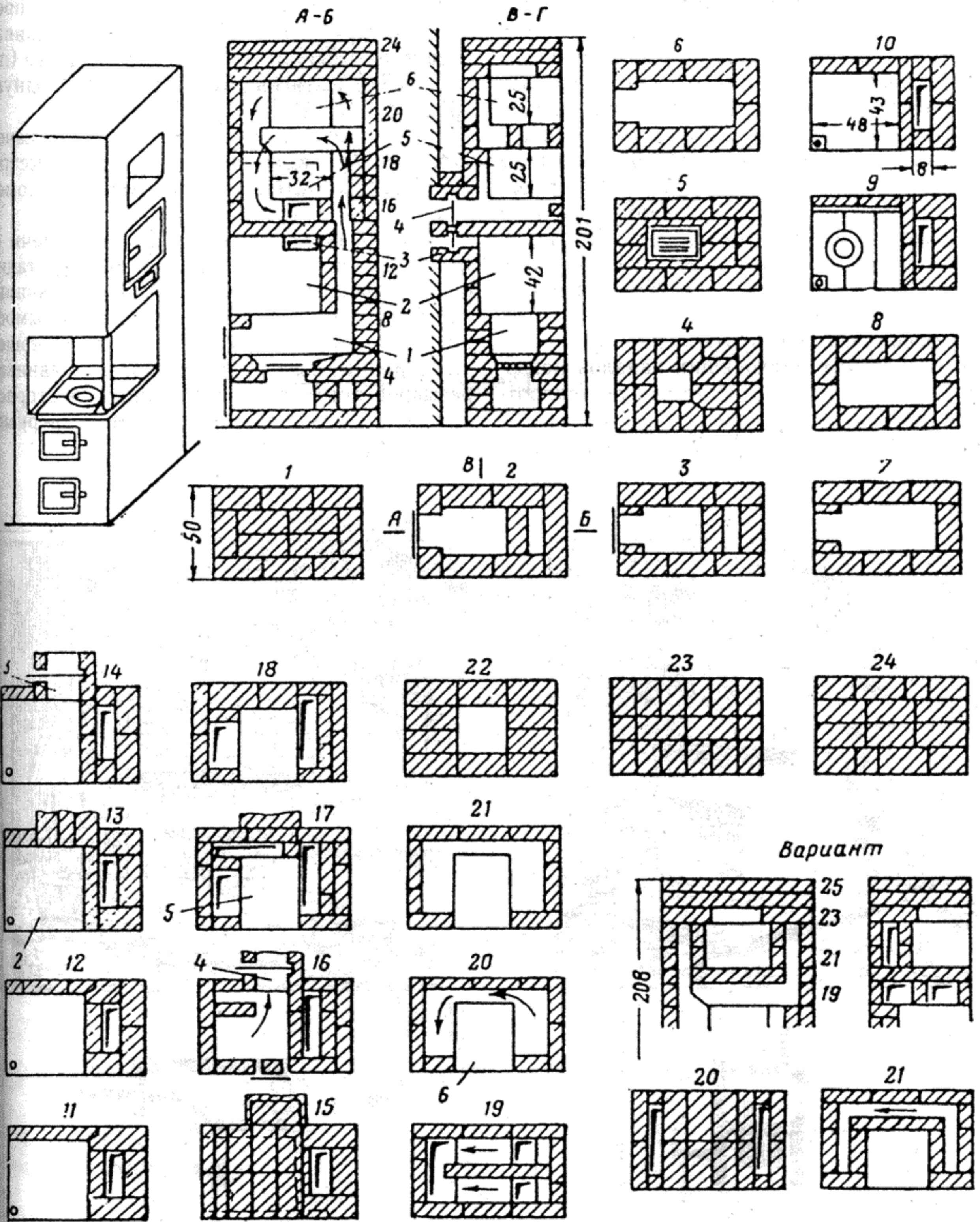
Малогабаритная отопительно-варочная печь Укргипросельстроа: 1 — топка; 2 — варочная камера; 3 — отверстия для вытяжки из варочной камеры; 4 — патрубок; 5 и 6 — духовка
