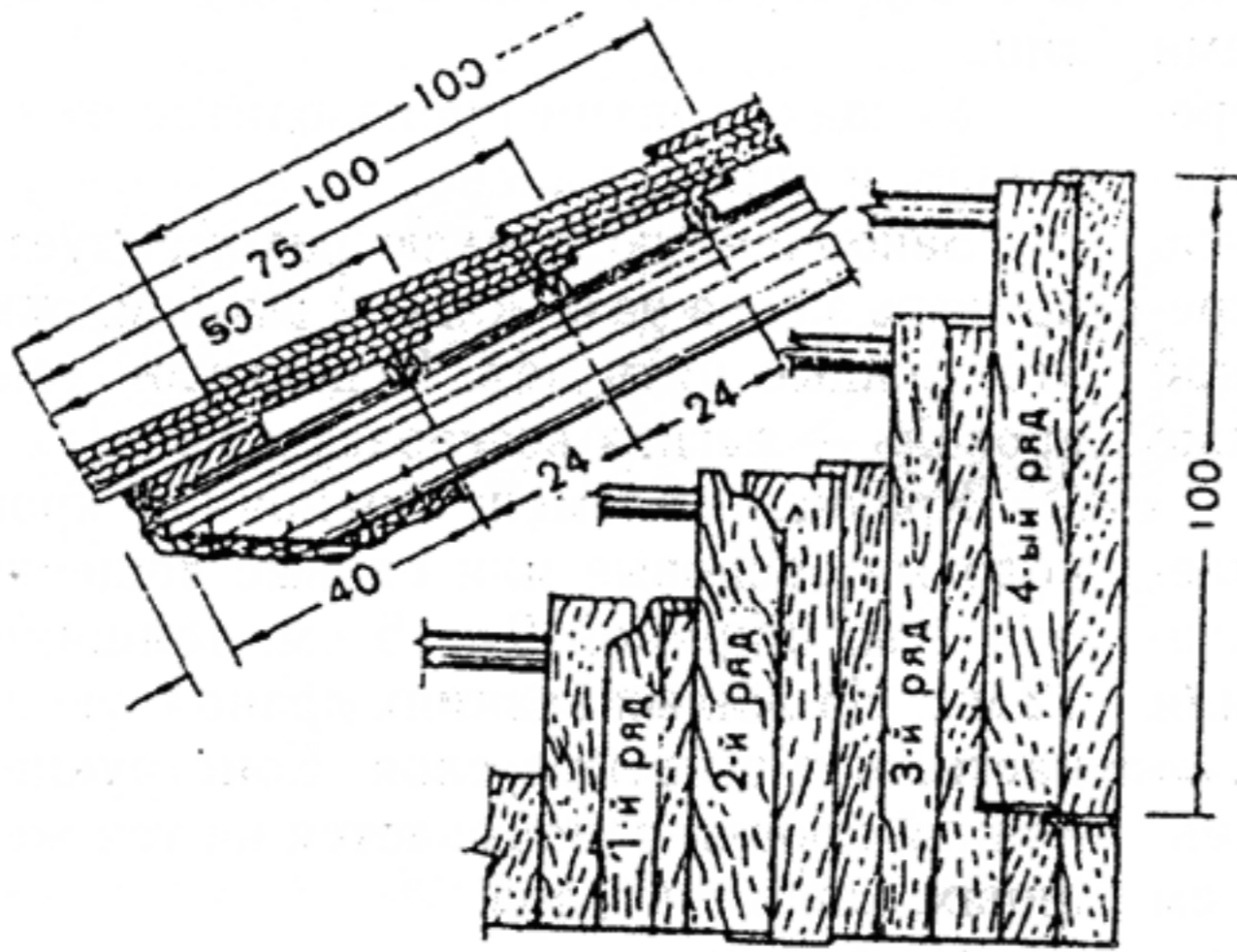
Драничная кровля
