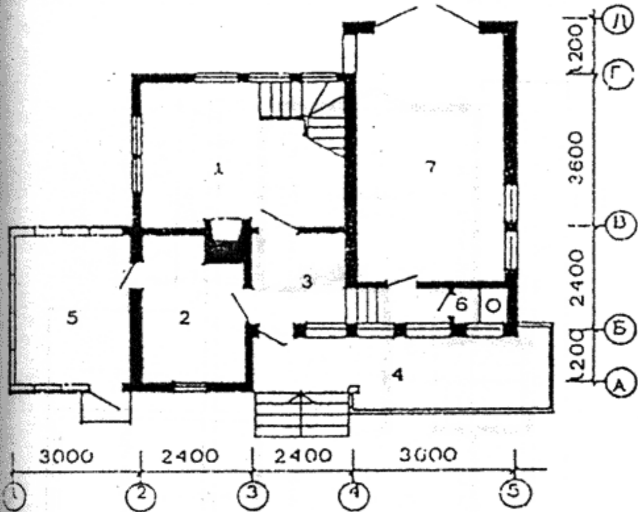
План этажа
