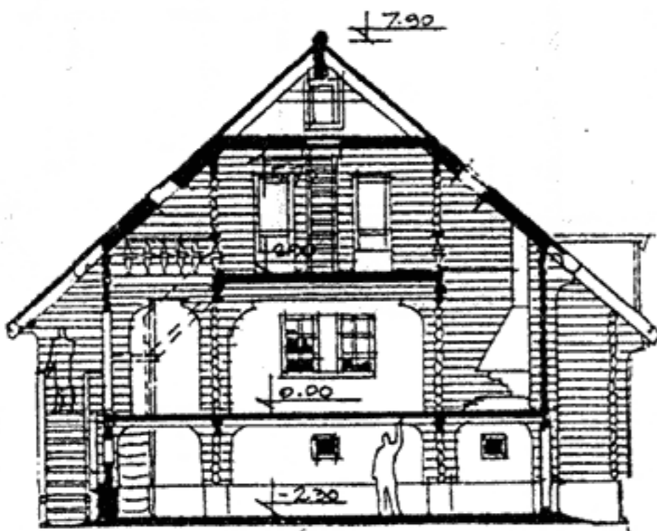
Разрез
