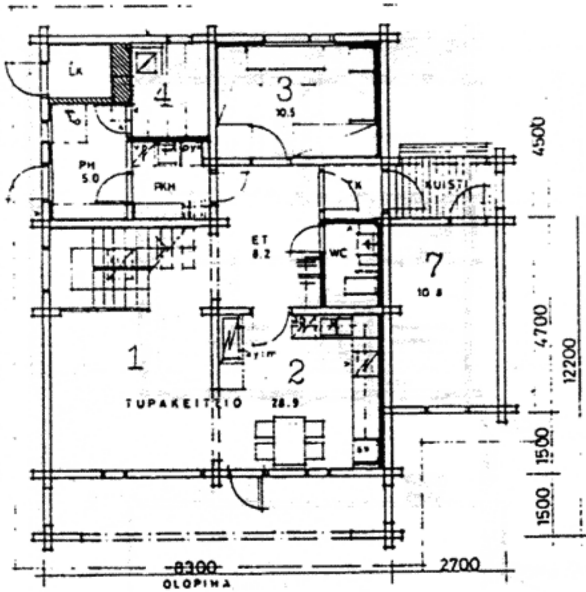
План I этажа
