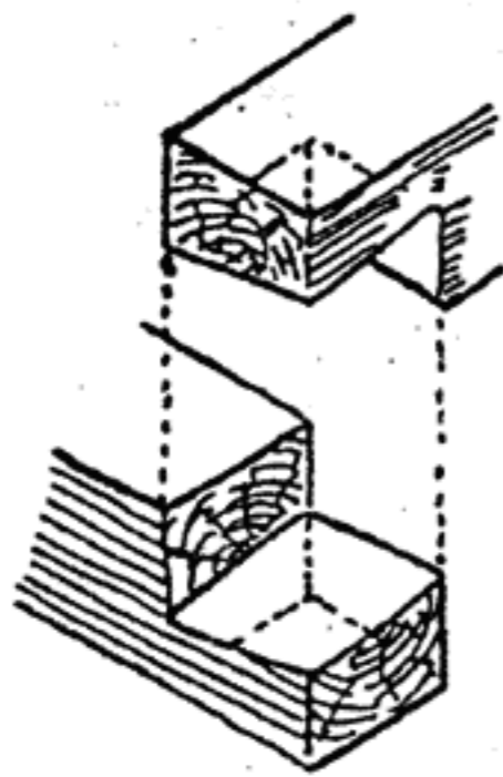
Замок в половину лапы
