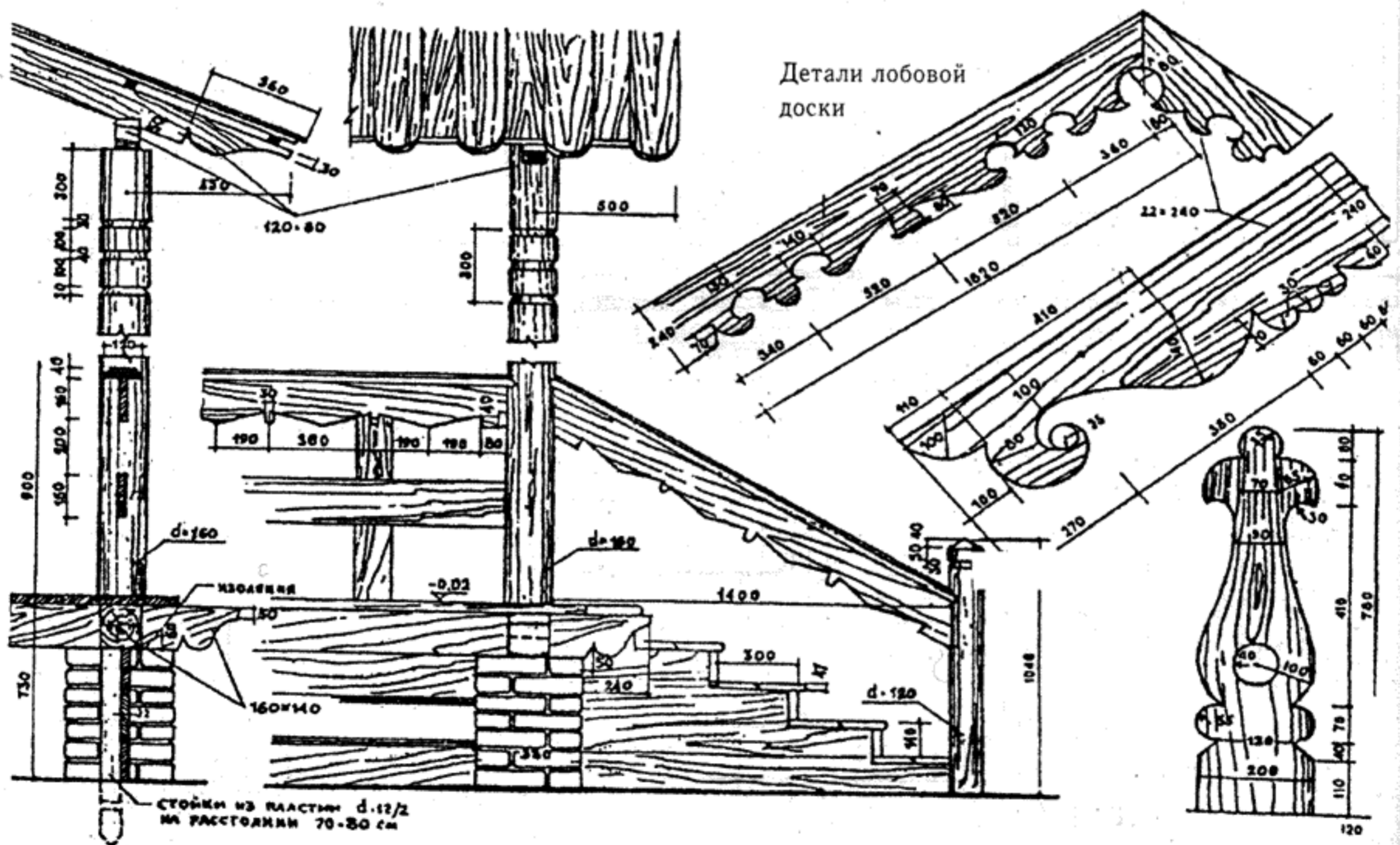
Детали крыльца
