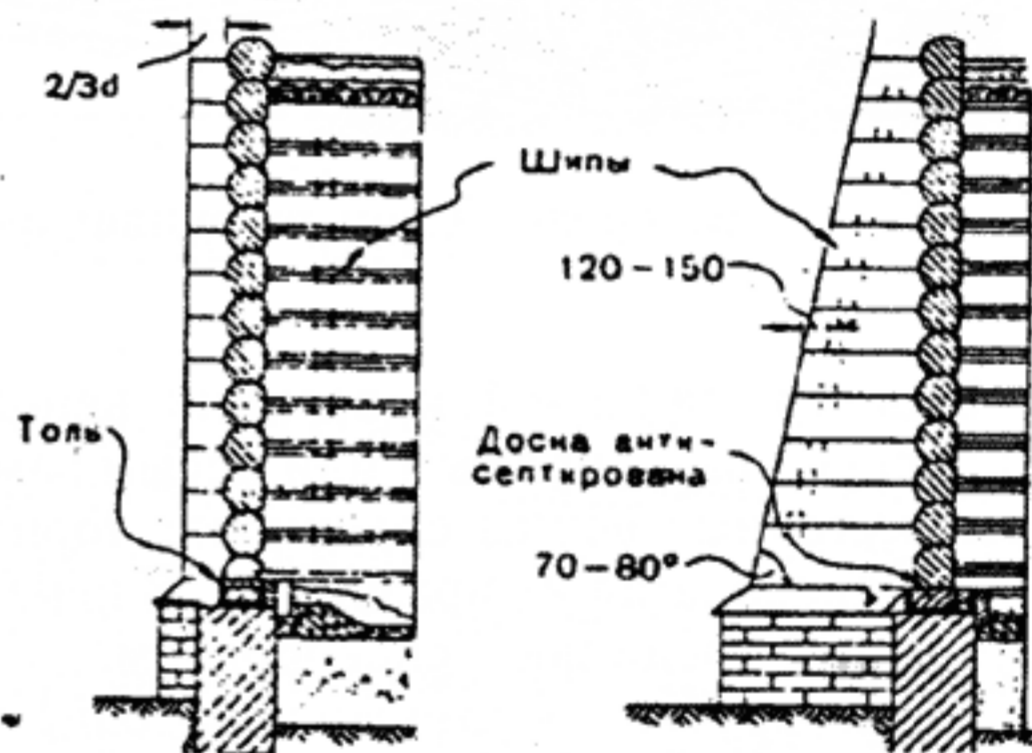
Коротыши
