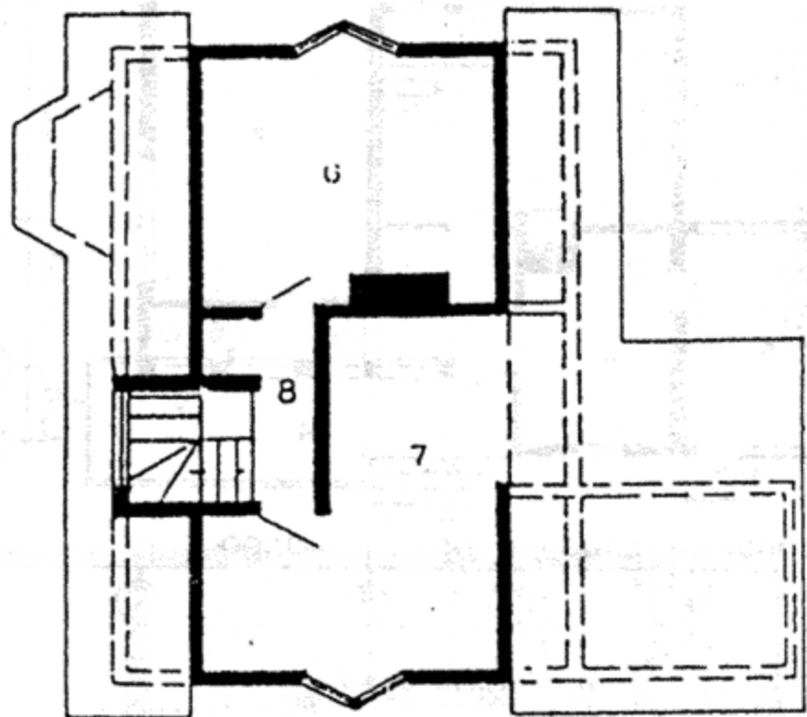
План мансарды
