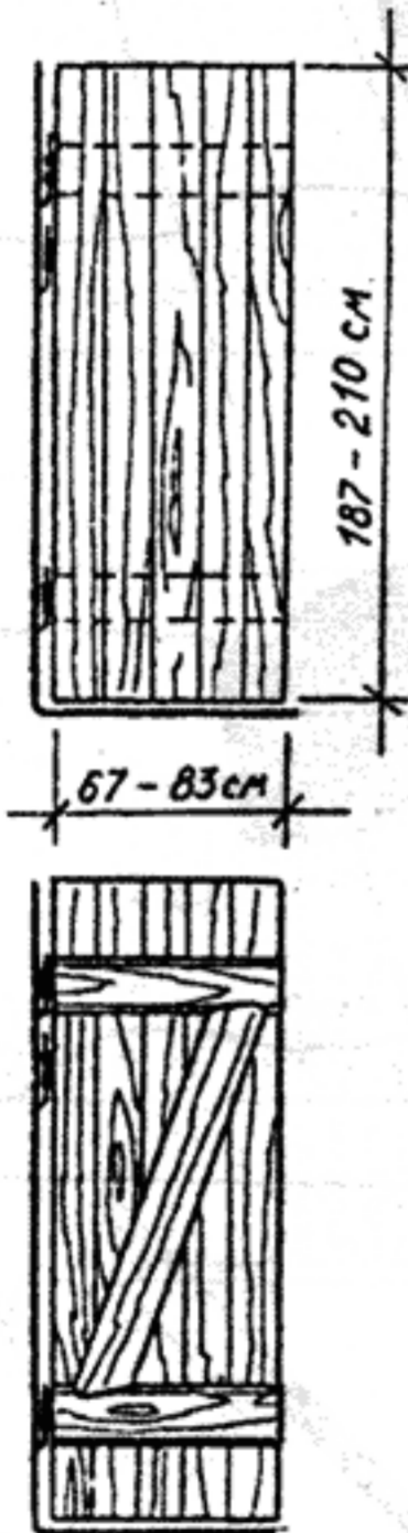
Дверь сарайная
