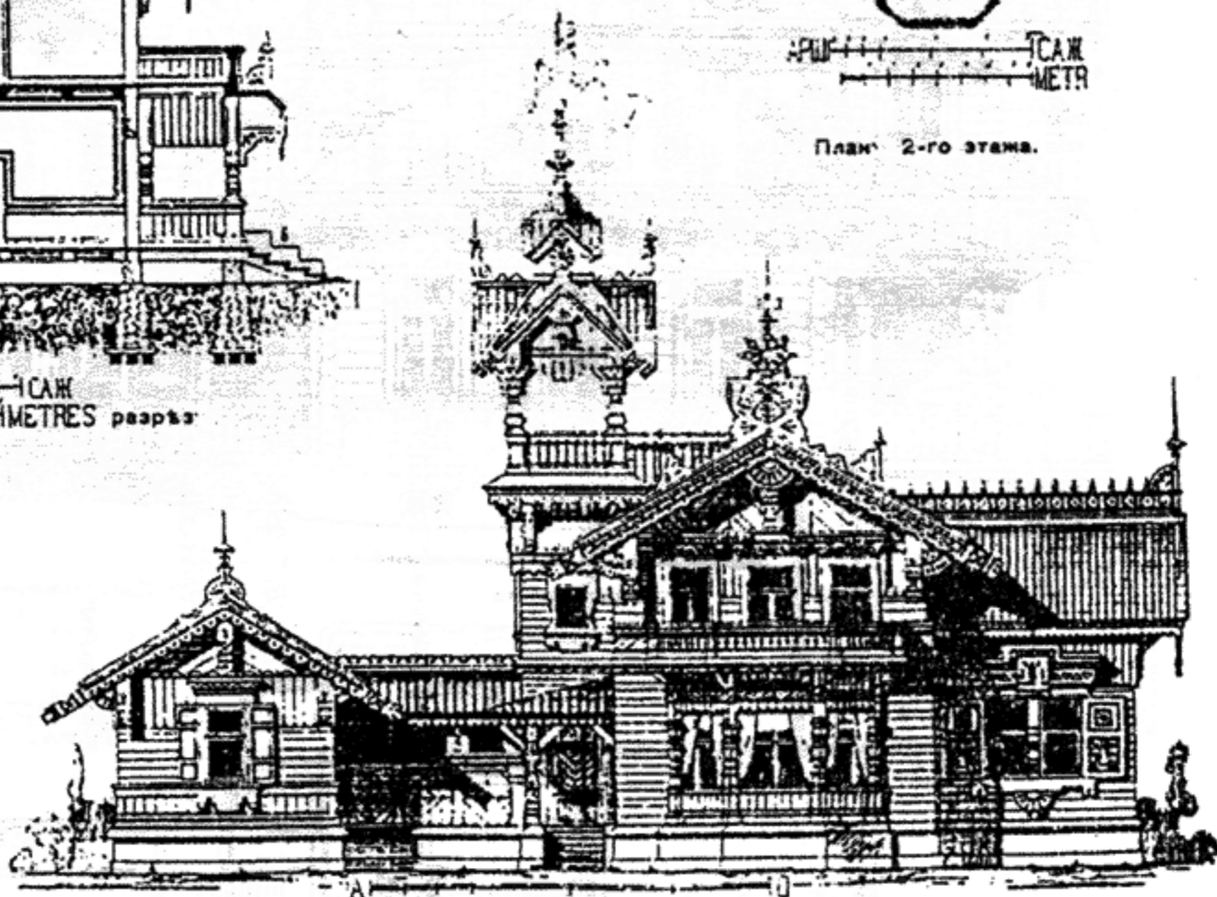
Главный фасад
