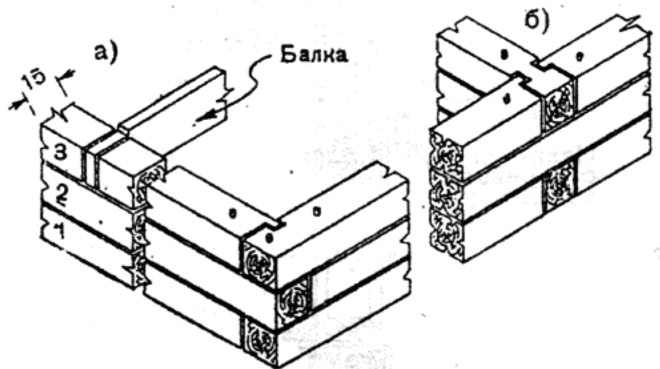
Рубка брусчатых стен
