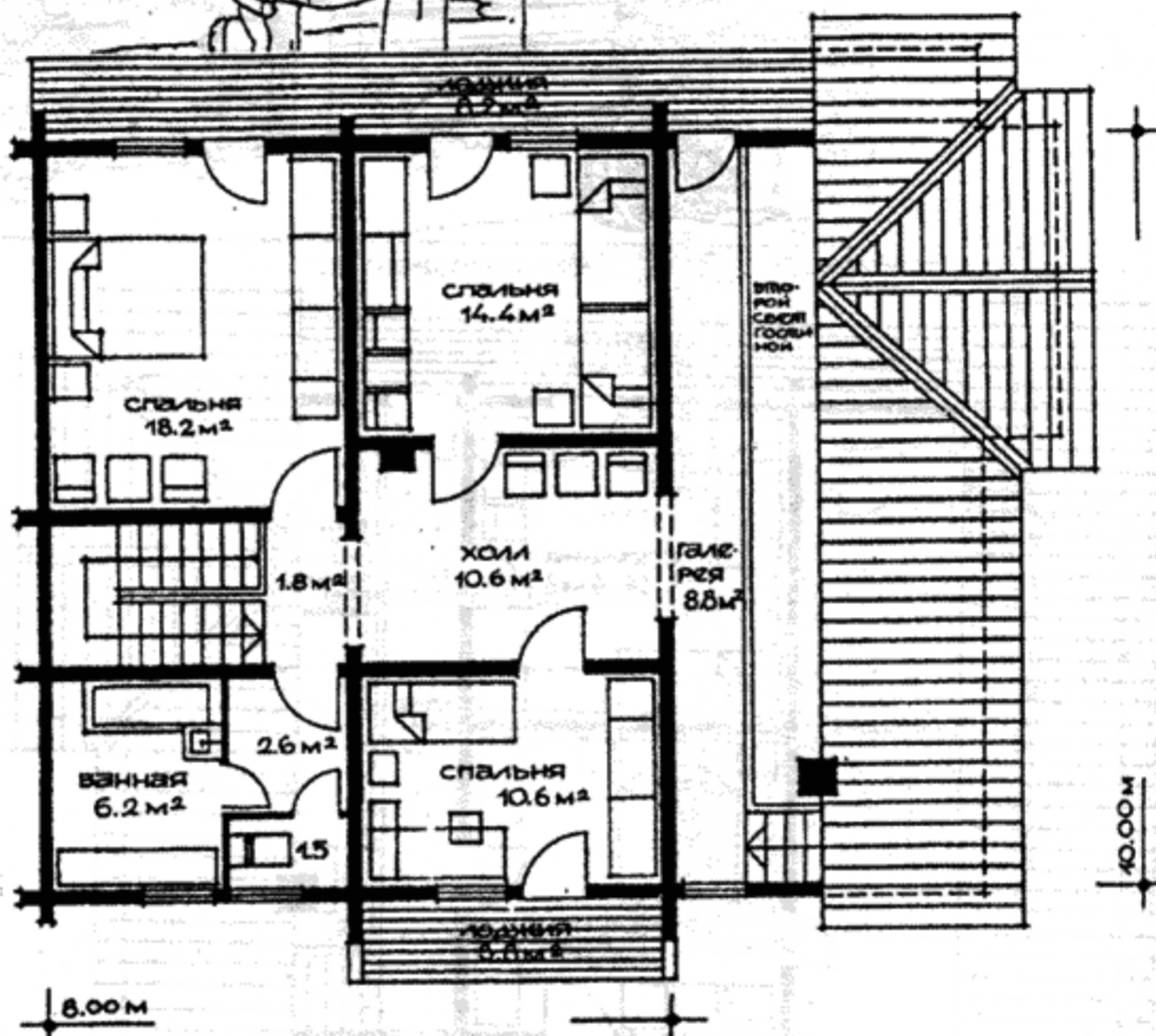
План 2 этажа
