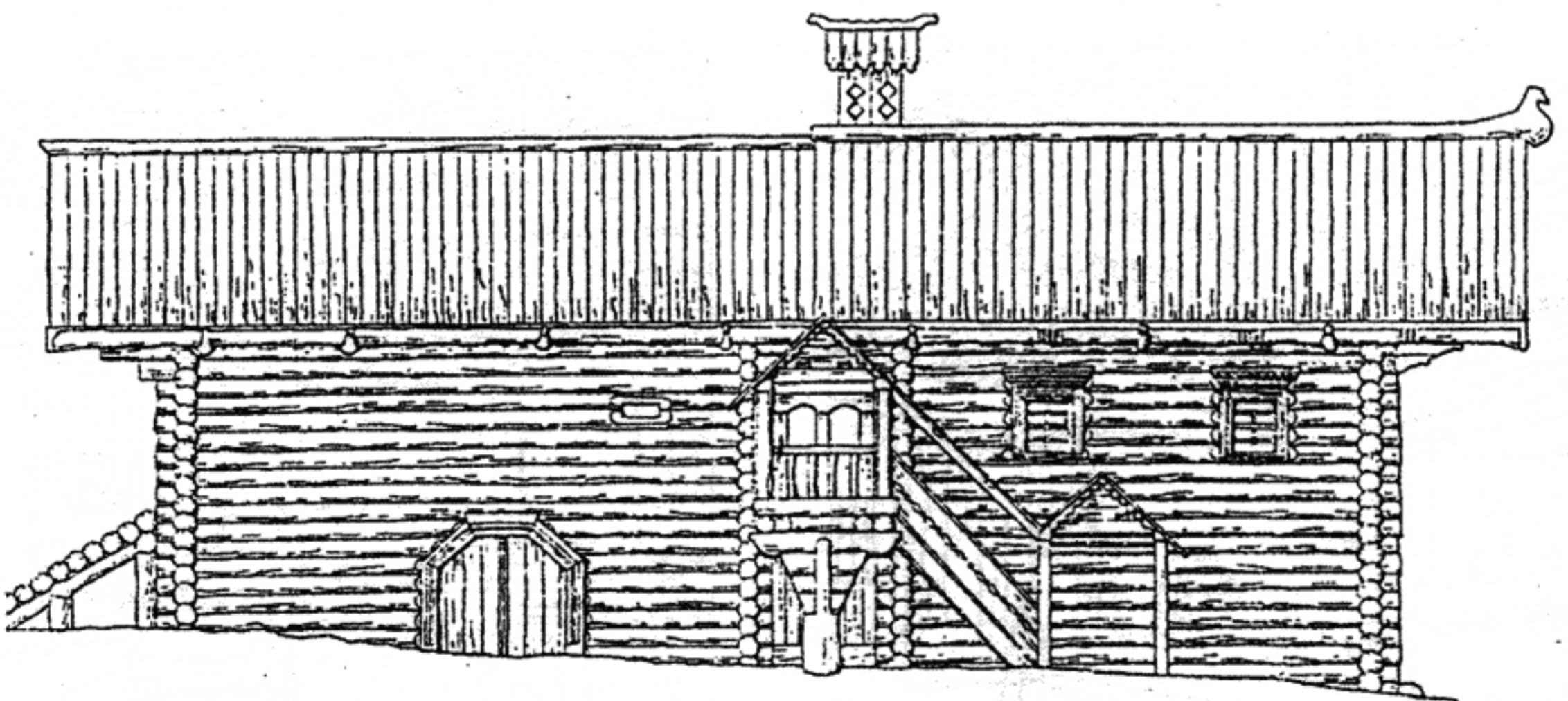
Боковой фасад
