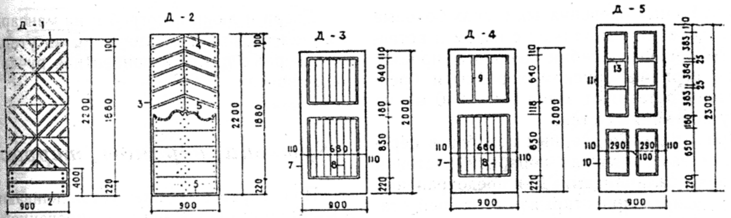
Двери наружные
