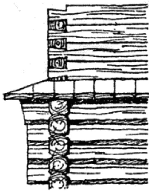
Рубка угла
